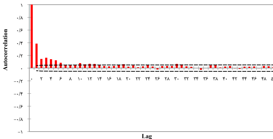
شکل ۳. نمودار ACF در سری زمانی بازدهی روزانه شاخص کل بورس اوراق بهادار تهران
