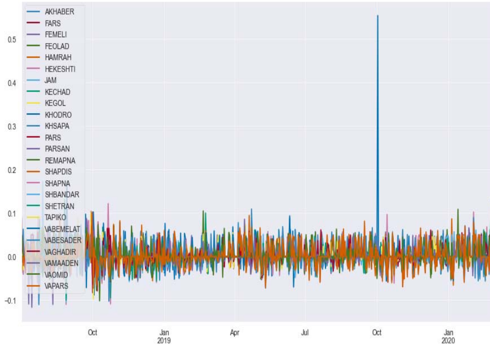
شکل ۷. بازده سهام
