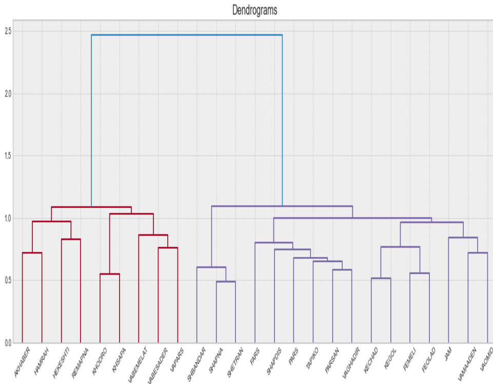
شکل ۸. دندروگرام
