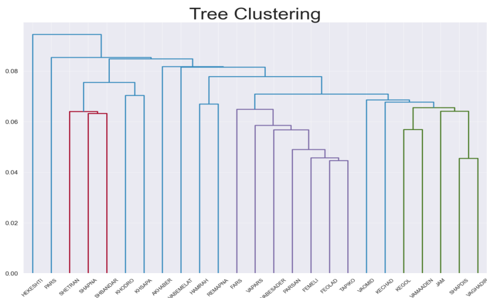
شکل ۴. نمودار خوشه‌بندی
